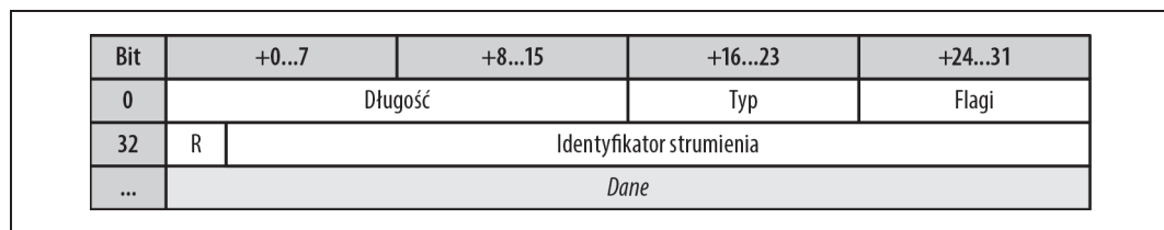
Rysunek 12.6. Jednolity 8-bajtowy nagłówek ramki
