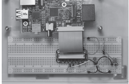
RYСУNEK 3.8. Gotowy obwód testowy z przyciskiem
