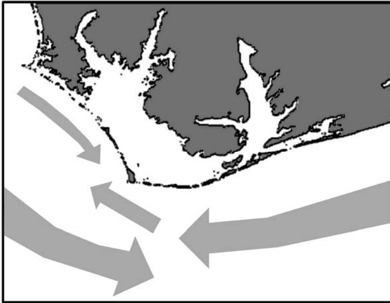
Rysunek 1.3. Prądy morskie w pobliżu Przylądka Python
