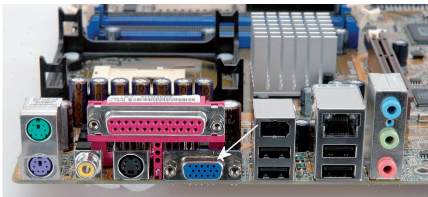
Rysunek 7.7. Przykład karty graficznej zintegrowanej z płytą główną
