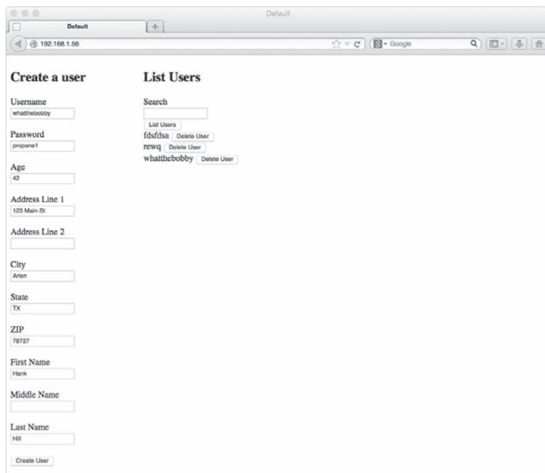
Rysunek 2.7. Aplikacja CsharpVulnJson otwarta w przeglądarce Firefox
